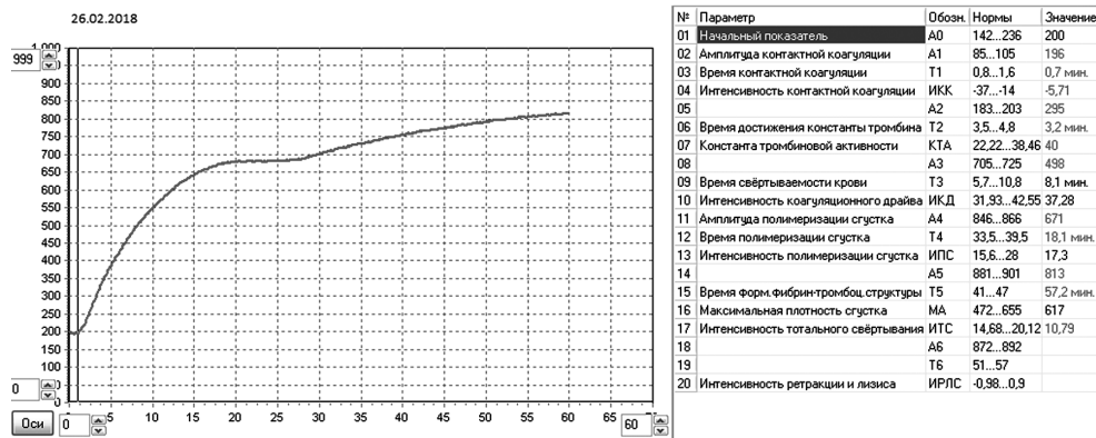
Мал. 4. Тромбоеластограма НПТЕГ з таблицею параметрів
